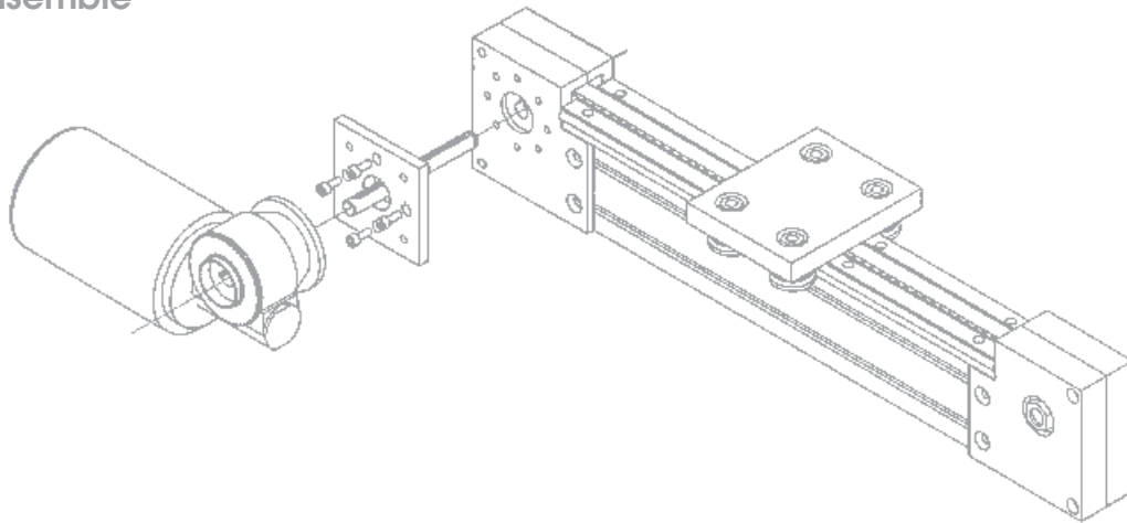
BRIDE D'ADAPTATION CARREE
